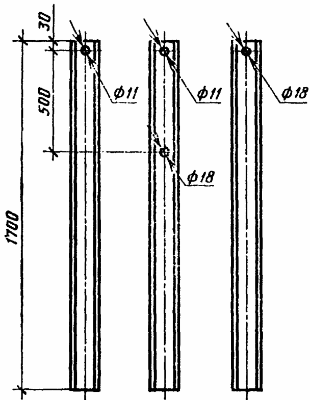
Стойки мостовые
