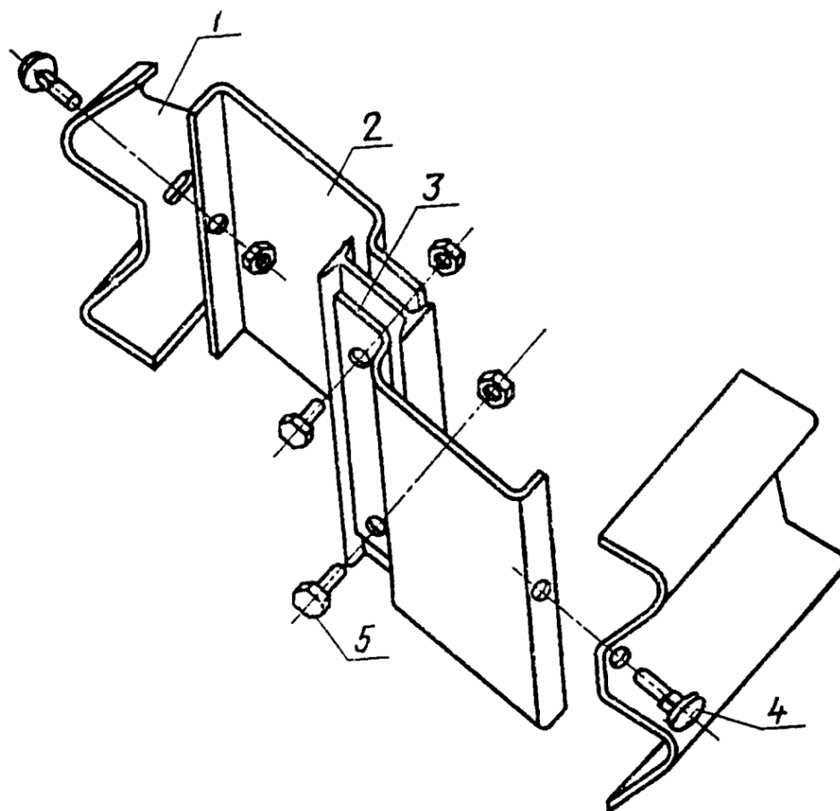
1 - балка; 2 - стойка; 3 - консоль-амортизатор; 4 - болт М16 х 45.58 ГОСТ 7802-81; 5 - болт М16 х 1,5-8г х 30.58 ГОСТ 7798-70
