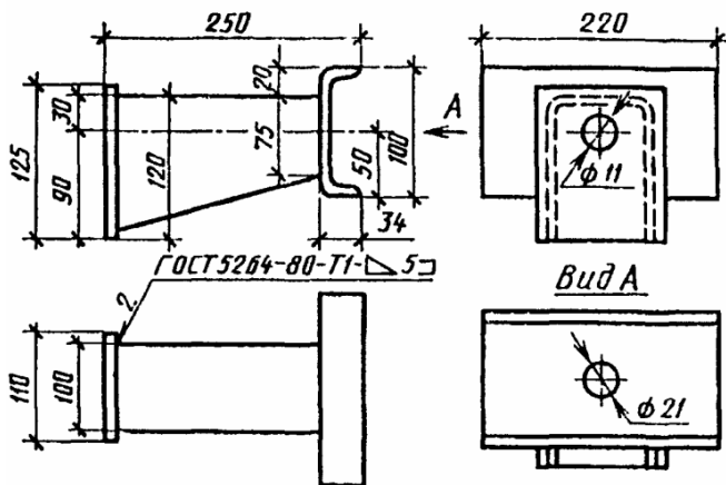
Консоль-распорка - КР
