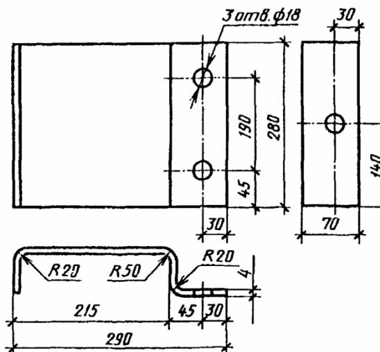
Консоль - амортизатор - КА
